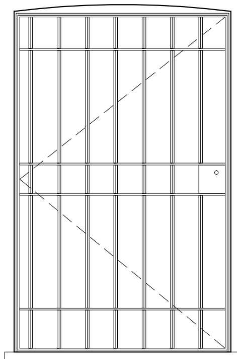
se.6 portafinestra camera 1B dim. vano luce cm 114x182h telaio fisso piatto 40x10 telaio mobile piatto 30x10; quadro 14x14 peso kg 58,000 circa
