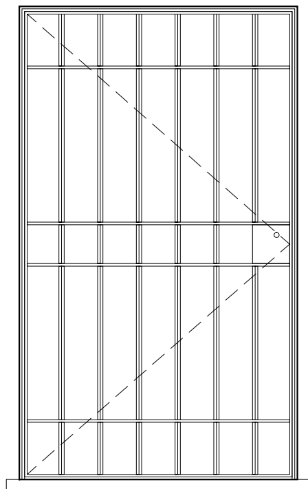
se.5 portafinestra camera 1A dim. vano luce cm 107x182h telaio fisso piatto 40x10 telaio mobile piatto 30x10; quadro 14x14 peso kg 51,000 circa
